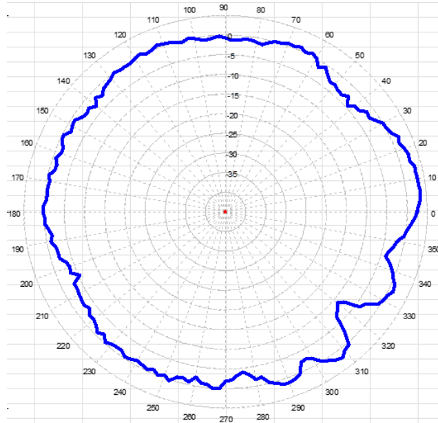
2.45 MHz
