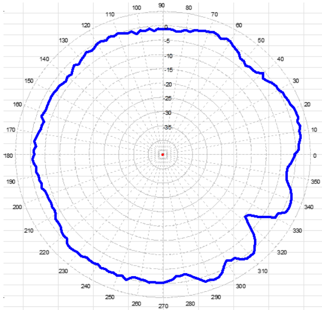
2.4 MHz
