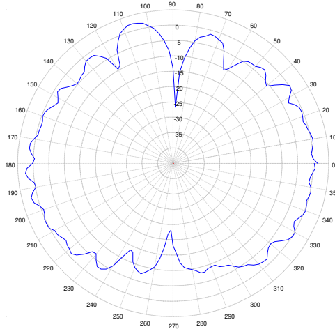
4900 MHz. ELEVATION
