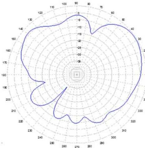
2.45 GHz. ELEVATION
