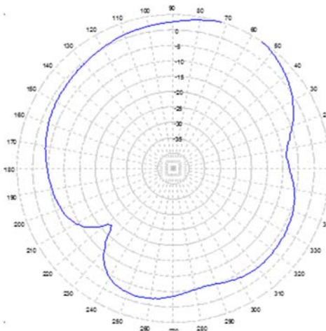
2.45 GHz. AZIMUTH
